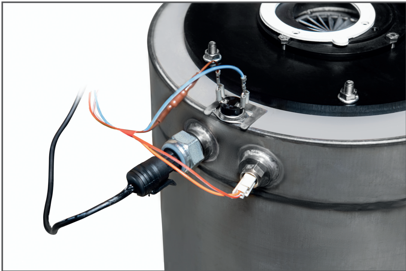
Реле давления, предохранительный термостат и датчик температуры
