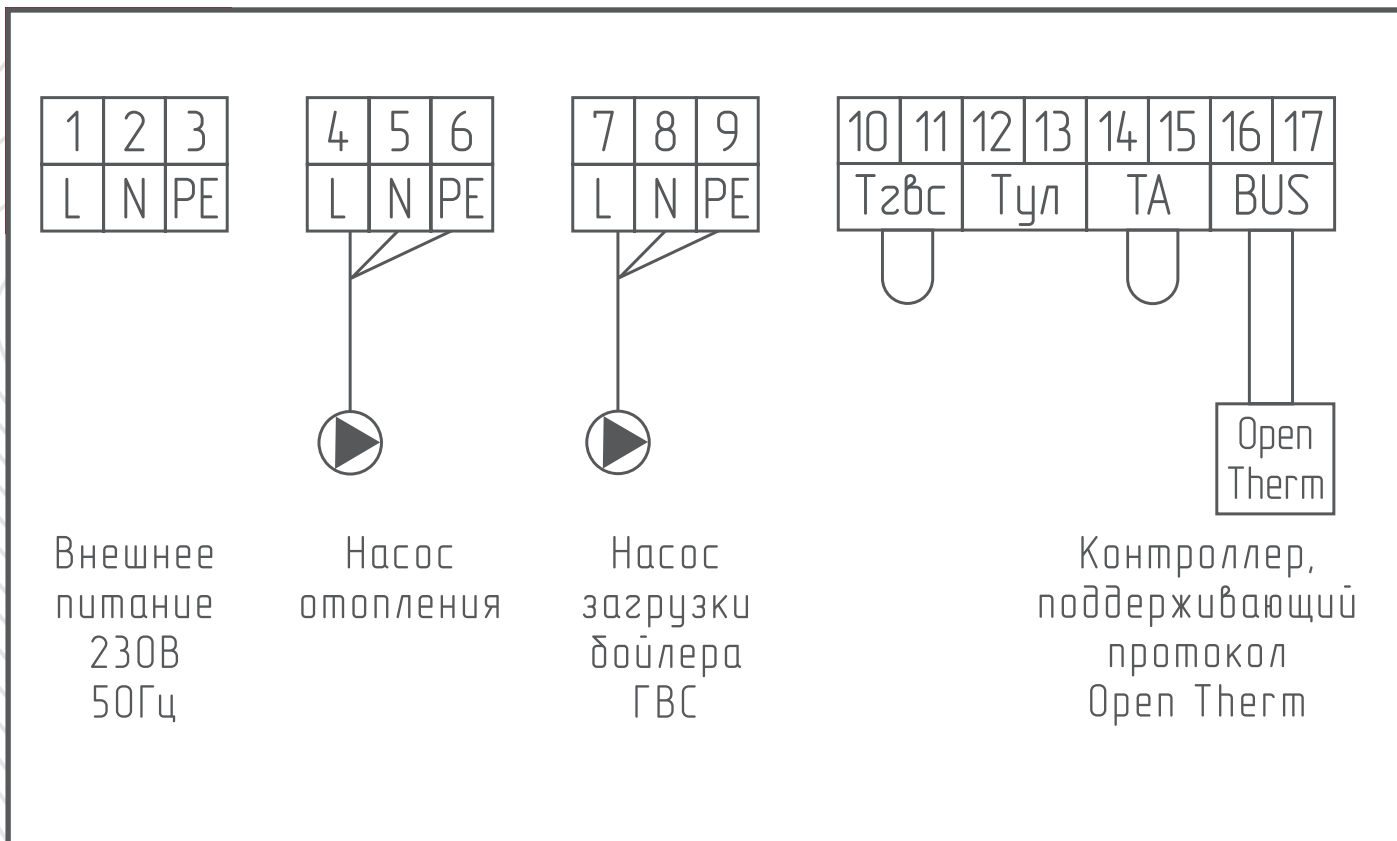
Клеммная плата
