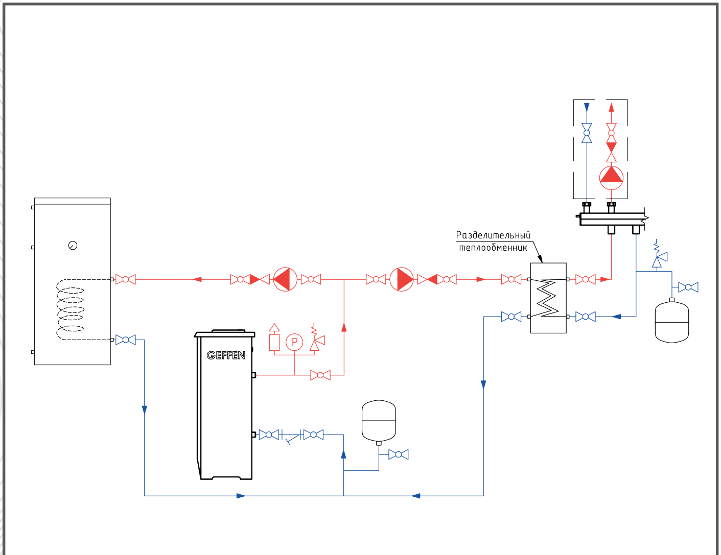
Схема подключения котла в существующую/реконструируемую систему отопления
